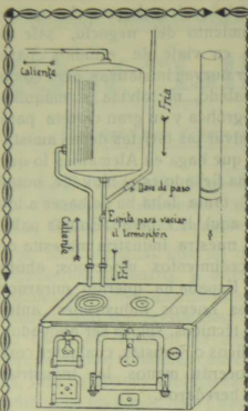
Esquema de una cocina provista de termosifón de cobre
