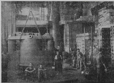
Turbina nitradora para la fabricación de explosivos
